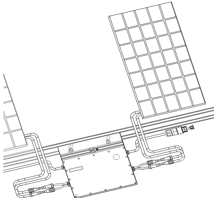
Fig.1 Posição de instalação do microinversor
